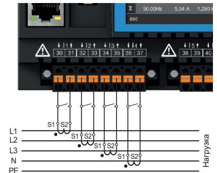
Рис. Пример подключения «Измерение тока»
