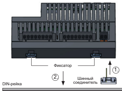
Рис. Устройство с шинным соединителем на DIN-рейке
