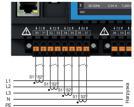
Рис. Пример подключения «Измерение тока»
