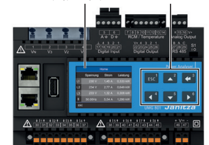
Рис. Стандартная индикация UMG 801-PA – Значения измерения
