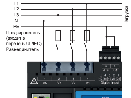
Рис. Пример подключения «Измерение напряжения»
