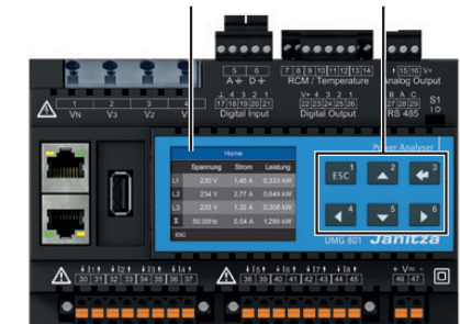
Рис. Стандартная индикация UMG 801-PA – Значения измерения
