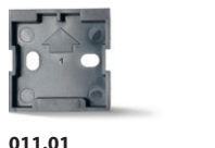
Адаптер для установки на панель (для типа 22.34), пластик, ширина 35 мм 011.01
