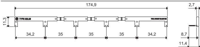
6-ти полюсный шинный соединитель для Тип 22.34, ширина 35 мм 022.26 (синий)
